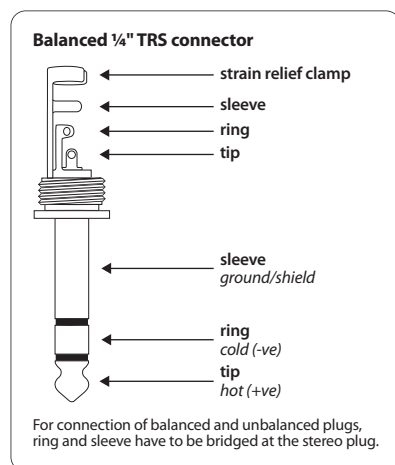
Fig. 4.2: Jack estéreo de 6,3 mm
