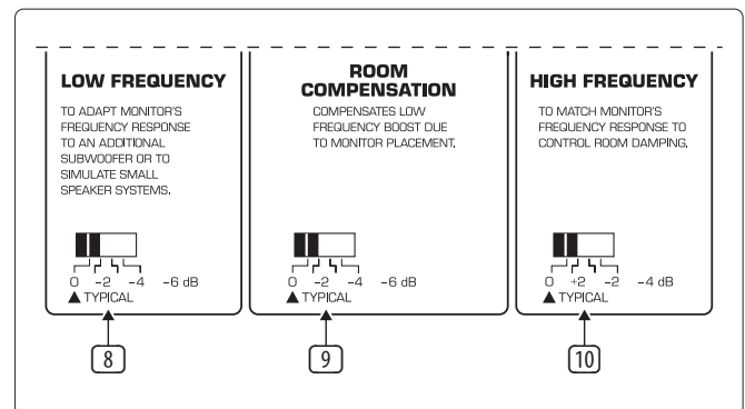
Fig. 2.5: Los elementos de mando del lado posterior del TRUTH
