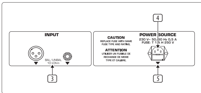
Fig. 2.2: Las entradas posteriores del TRUTH
