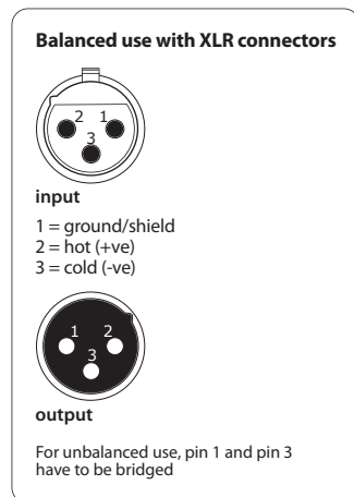
Fig. 4.3: Conexiones XLR
