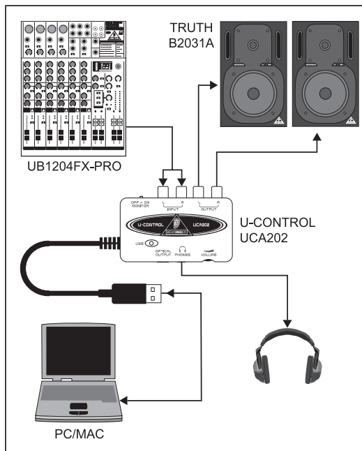
Fig. 4.1: Ejemplo de conexión usando la UCA202
